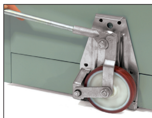
Anwendungsbeispiel
